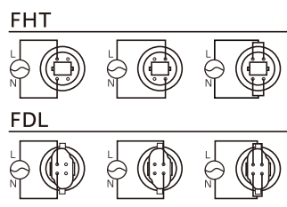
結線イメージ
