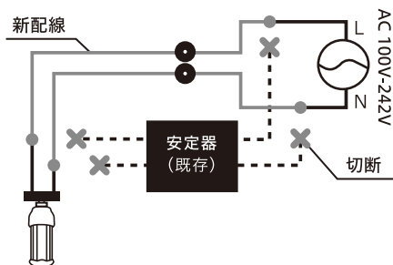
結線イメージ
